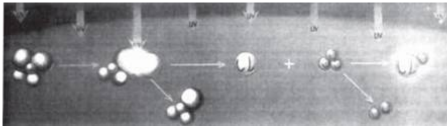
Fig. 3-5. Reacción del Ozono en moléculas.
